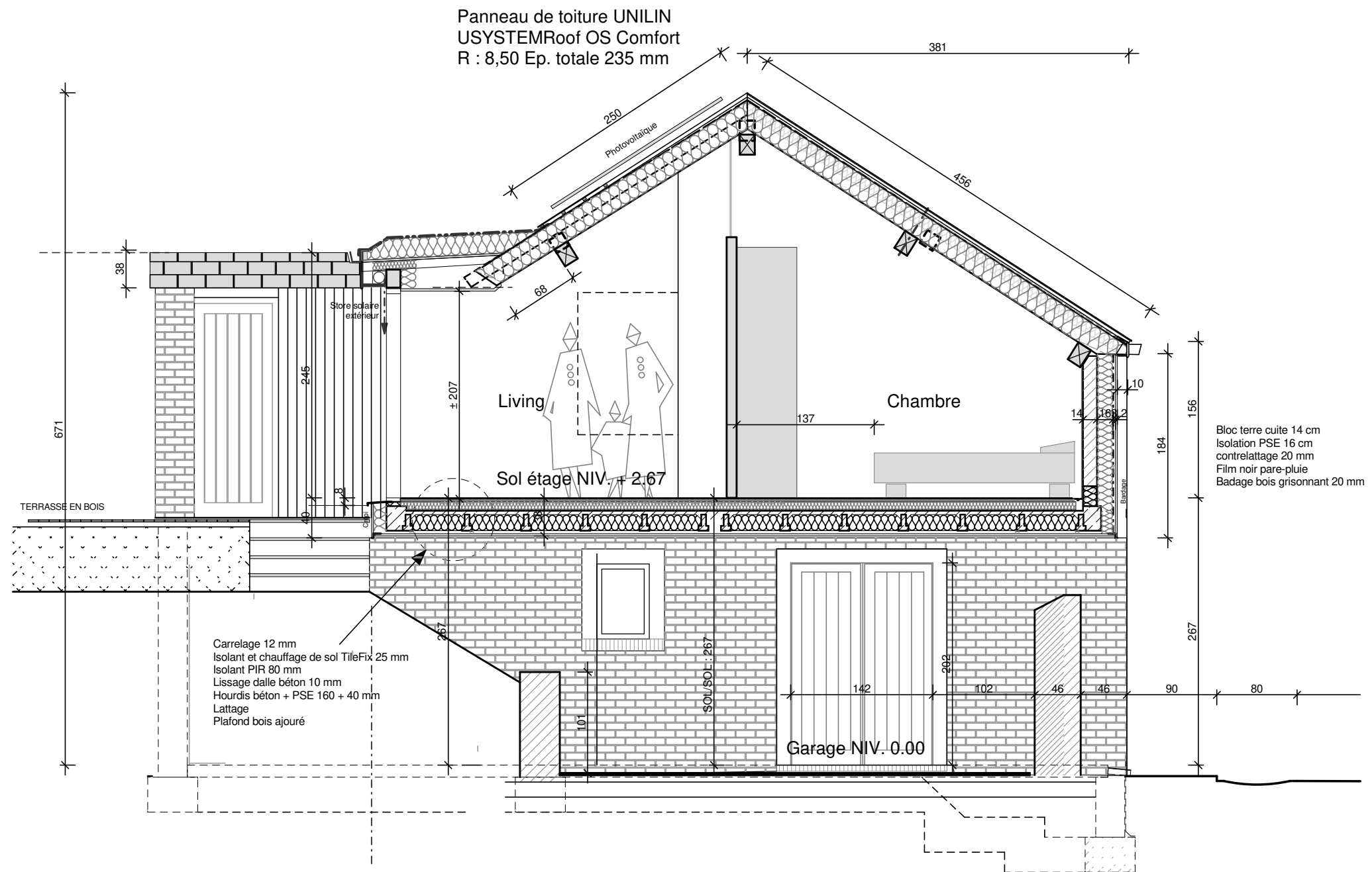
COUPE A dans l'extension
